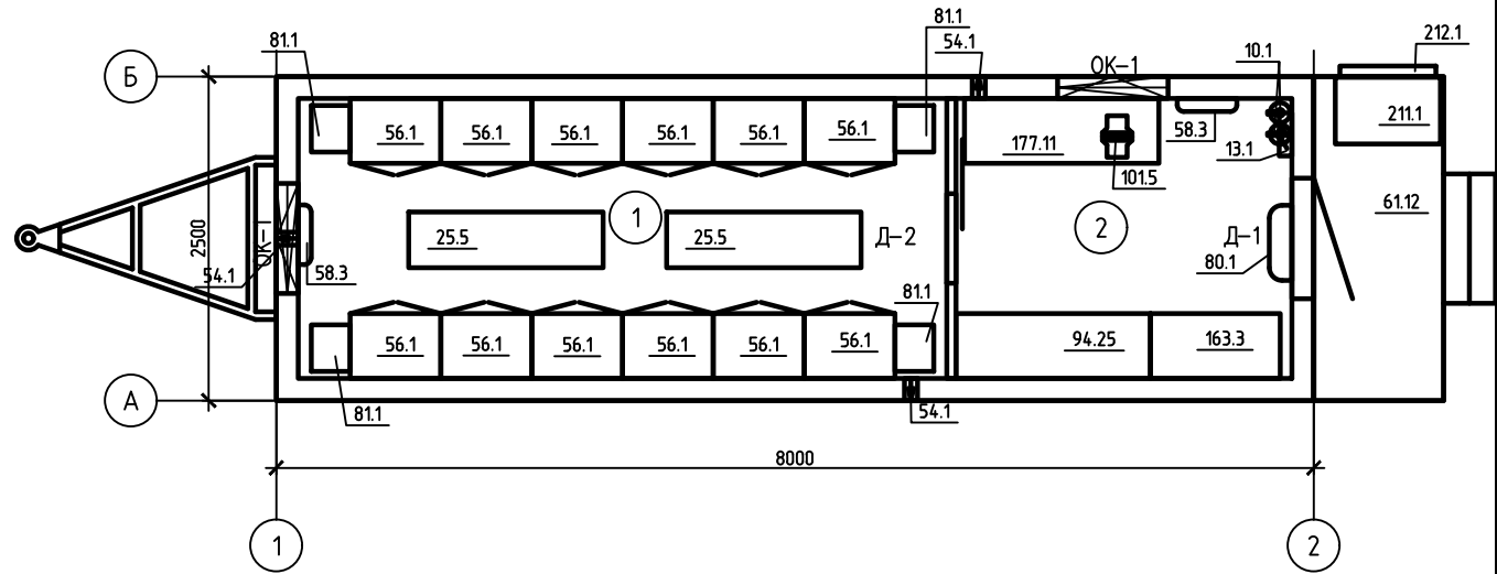
Схема расположения мебели и оборудования
